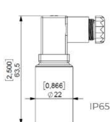
EN 175301-803-C
